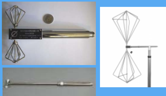
Biconicalアンテナ 20MHz~18GHz
